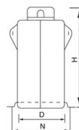
IP3906-XX (5000/5、5000/1) 产品侧视图
