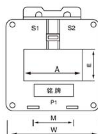
IP3906-XX (5000/5、5000/1) 产品正视图
