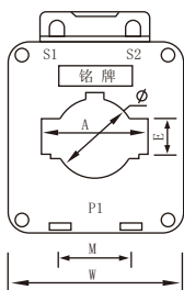
IP3906-XX (800/5、800/1、200/5、200/1) 产品正视图
